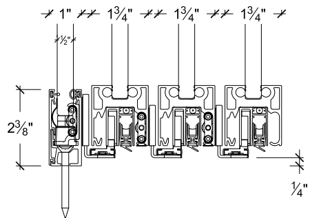
Single glazed in the open position Verre simple en position ouverte
