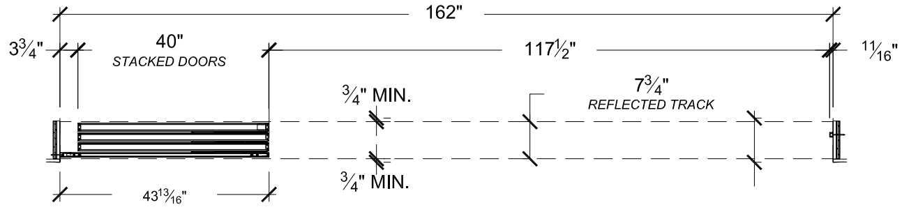
Example of a double glazed system on an opening of 162" in the open position Exemple d'un système sur une ouverture de 162 po avec verre double en position ouverte
