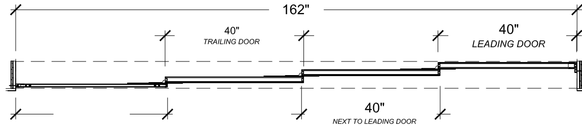
Example of a double glazed system on an opening of 162" in the closed position Exemple d'un système sur une ouverture de 162 po avec verre double en position fermée
