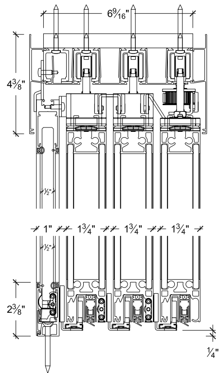
Double glazed in the open position Verre double en position ouverte
