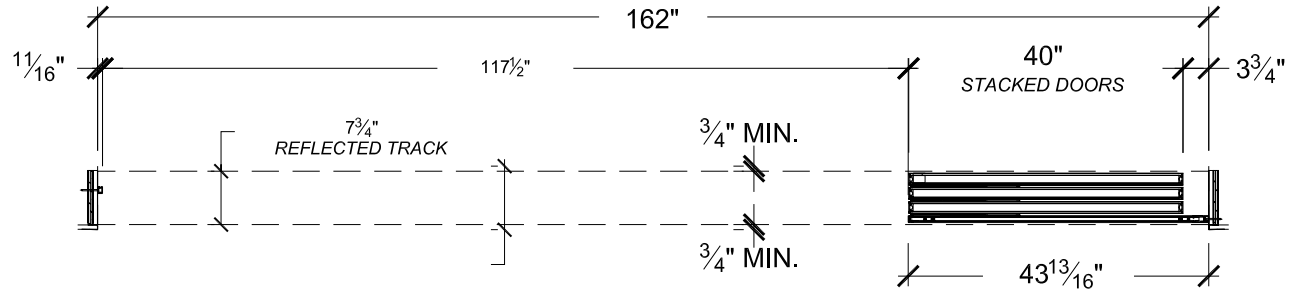
Example of a double glazed system on an opening of 162" in the open position Exemple d'un système sur une ouverture de 162 po avec verre double en position ouverte
