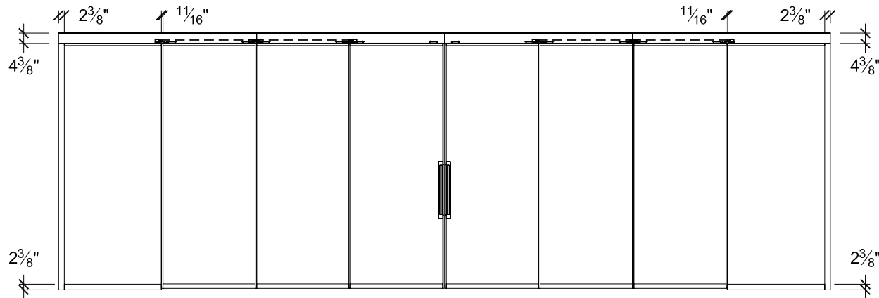
Single glazed left stacking and single glazed right stacking Empilage gauche verre simple et empilage droit verre simple
