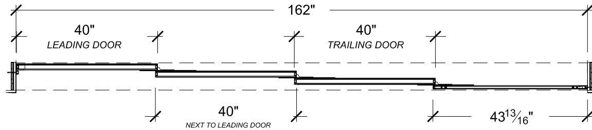
Example of a double glazed system on an opening of 162" in the closed position Exemple d'un système sur une ouverture de 162 po avec verre double en position fermée
